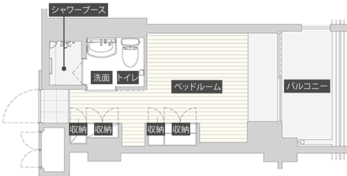
住室平面図
