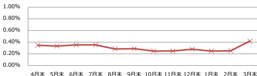
令和3年度のKKRの資産全体の推定トラッキングエラーの推移
